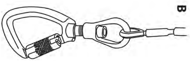
Figura 5: Inspección del mosquetón con indicador de carga
