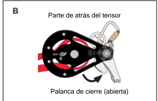
FIGURA 8 - REDUCCIÓN DE LA TENSION DE LA LÍNEA SALVAVIDAS
