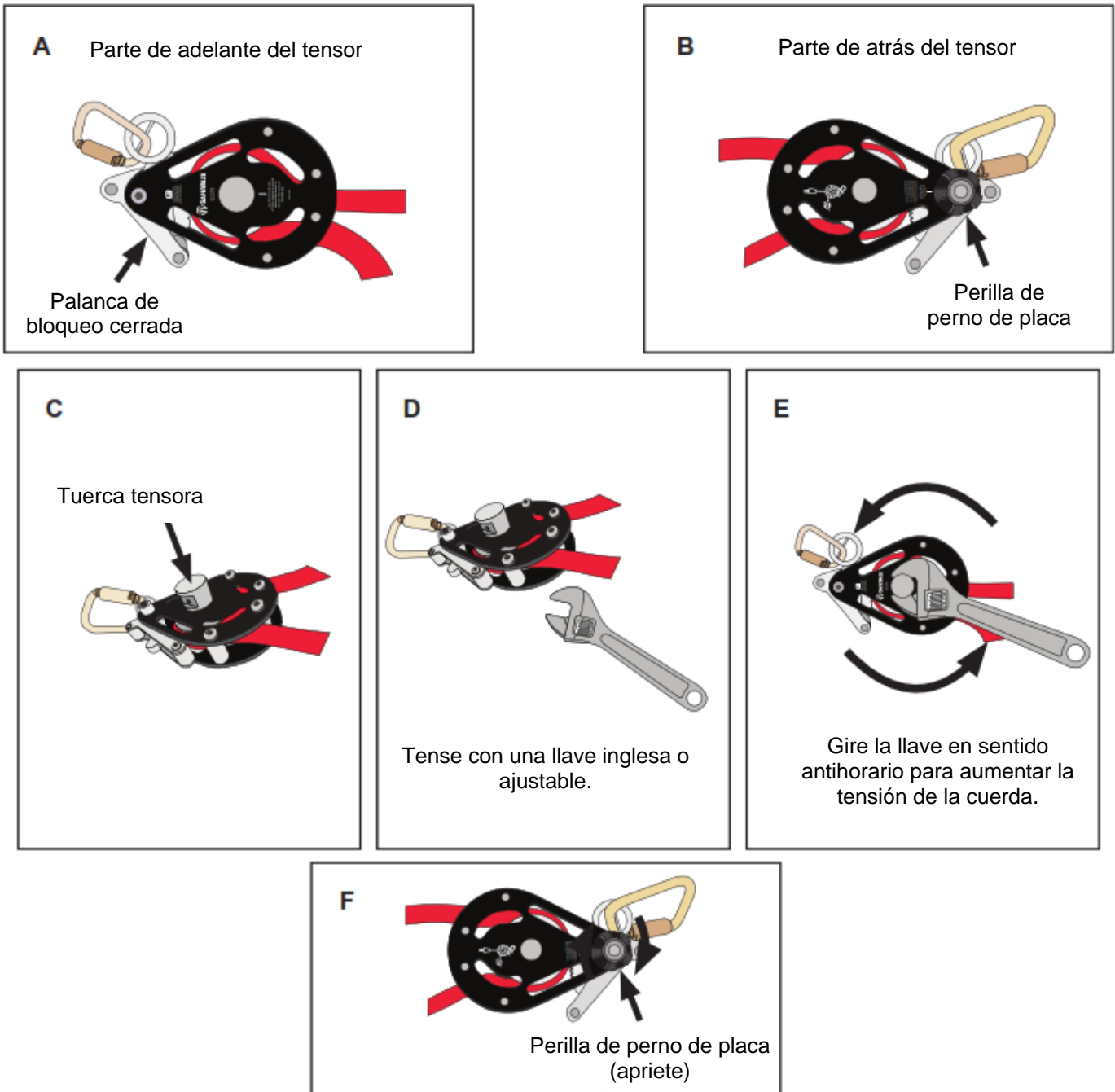
FIGURA 7 - FUNCIONAMIENTO DEL TENSOR DE CUERDA
