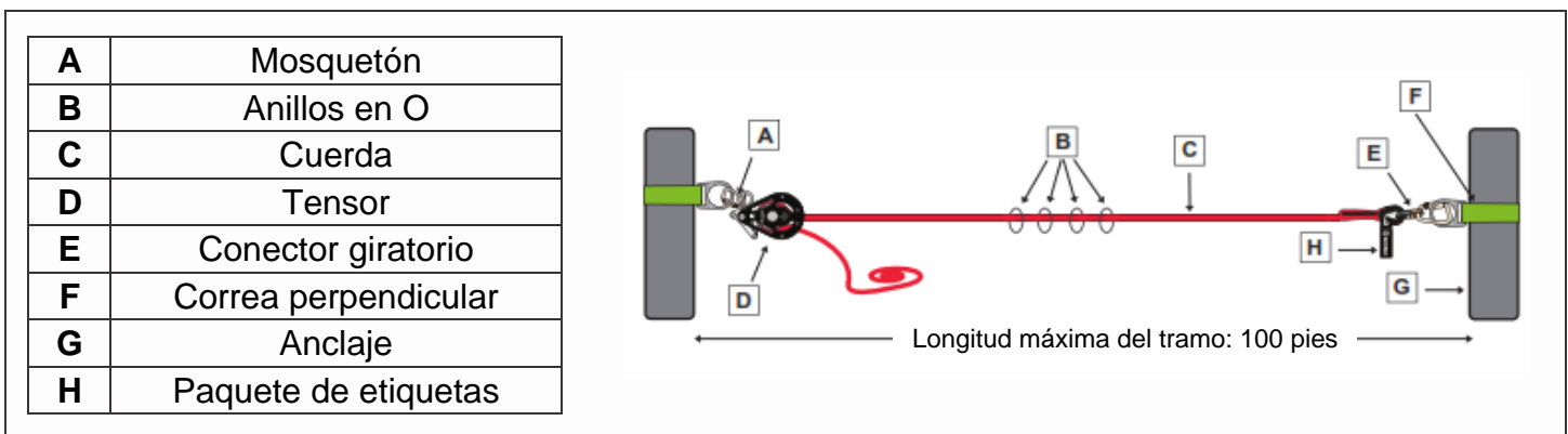
FIGURA 9 - COMPONENTES
