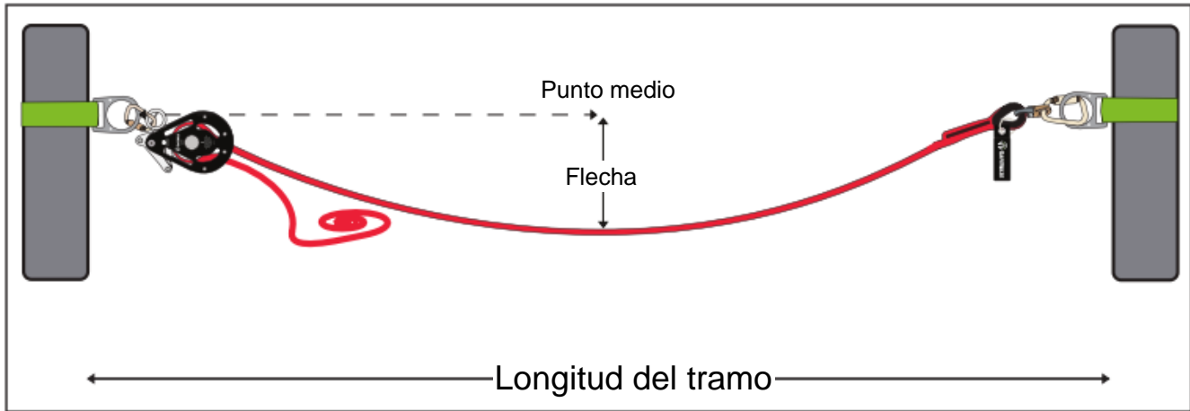
FIGURA 10 - FLECHAS DE LA HLL
