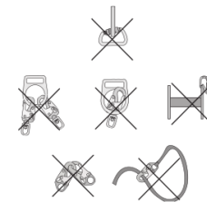
FIGURA 4 - CONEXIONES INCORRECTAS
