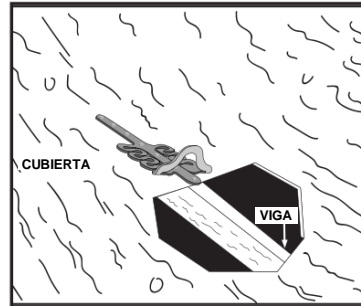
FIGURA 6 - VISTA SECCIONADA
