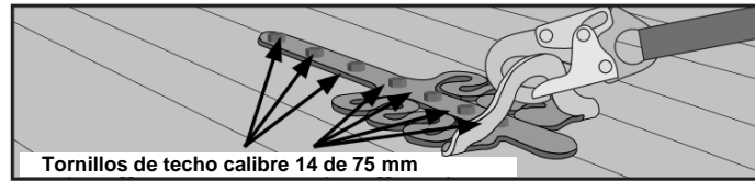
FIGURA 6 - INSTALACIÓN
